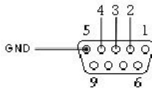
D-SUB 9ピン(メス)
